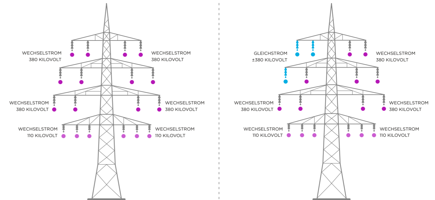
Beispielmast aus dem Teilabschnitt Rommerskirchen - Sechtem. Auch Strommaste anderer Bauart mit weniger Stromkreisen am Mast werden im Bereich zwischen Rommerskirchen und Landesgrenze NRW/RLP für die Gleichstromverbindung genutzt.
